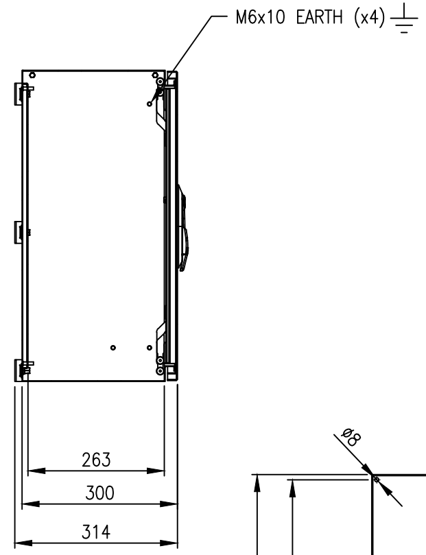
SECTION AV-AV
