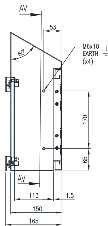
SECTION AV-AV
